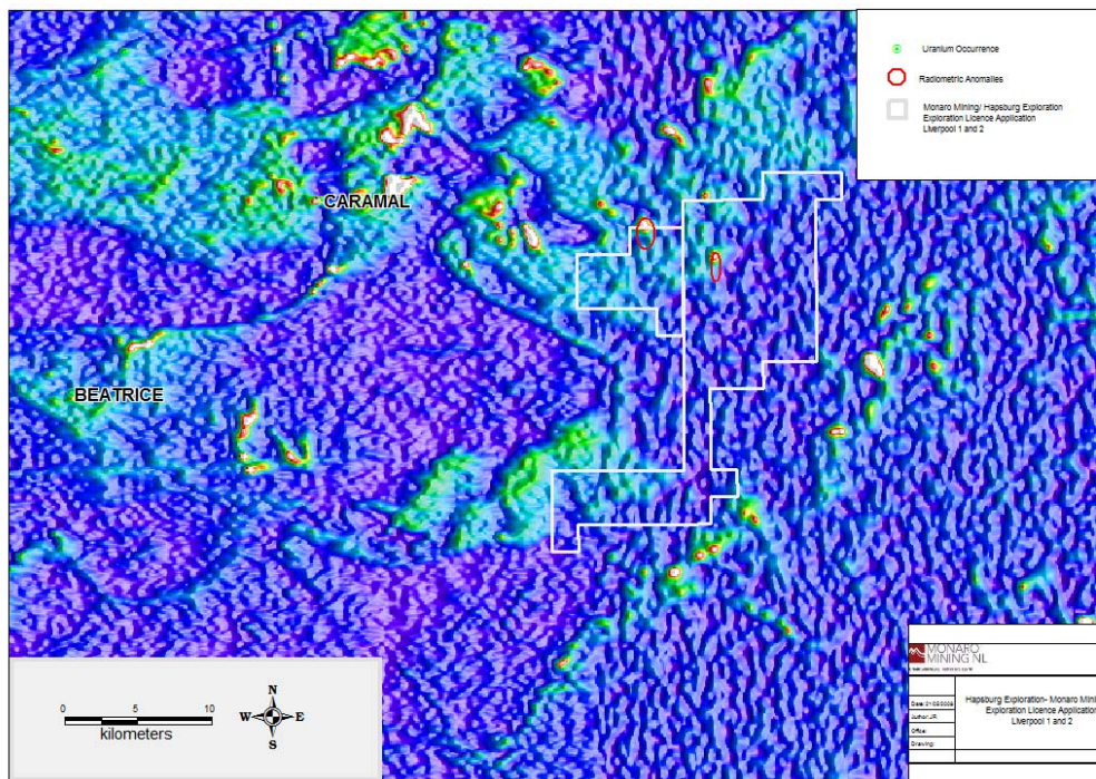
Abbildung 2: Regionale radiometrische Aufnahme mit Lage der Pachtgebiete Liverpool-1 und Liverpool-2. Man beachte die zwei Bullseye-Anomalien innerhalb von Liverpool-1 und Liverpool-2
