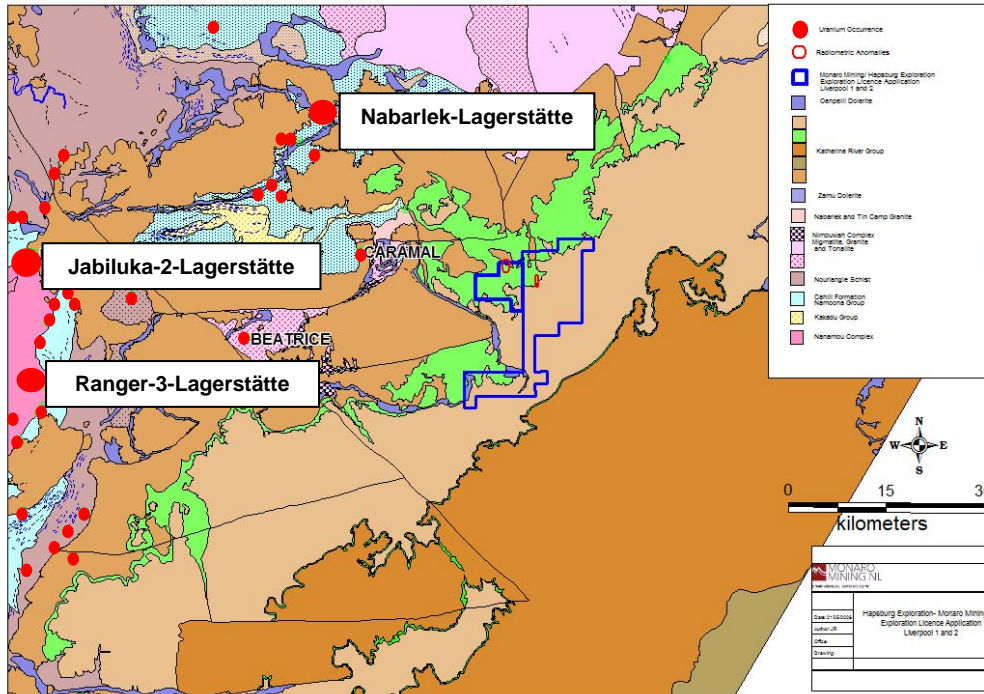
Abbildung 1: Lage der Pachtgebiete Liverpool-1 und Liverpool-2 mit regionaler Geologie und den in der Nähe befindlichen Uranlagerstätten
